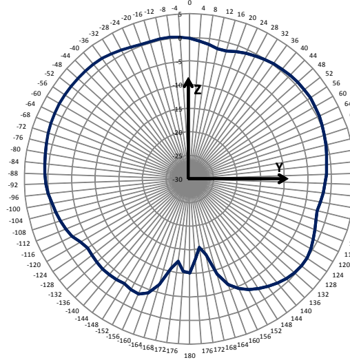
E-Plane
