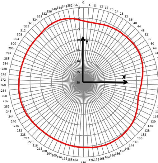
H-Plane
